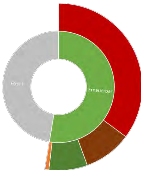
Wärmeerzeugung 2016 in %
