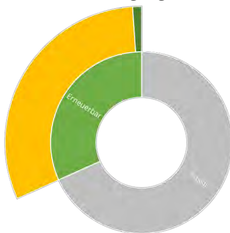
Stromerzeugung 2016 in %
