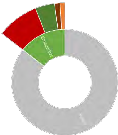
Wärmeerzeugung 2016 in %
