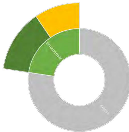
Stromerzeugung 2016 in %
