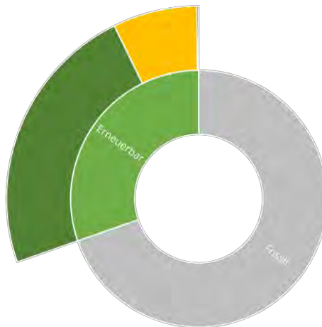
Stromerzeugung 2016 in %
