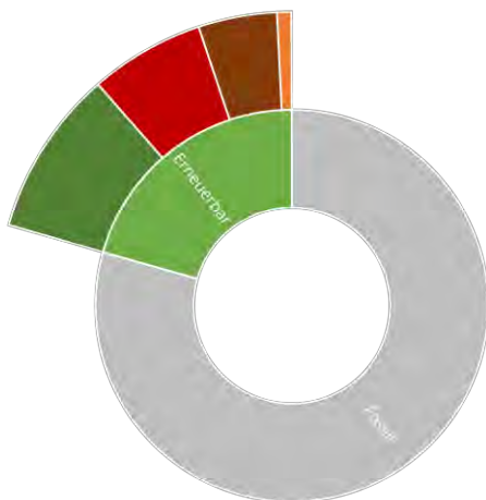
Wärmeerzeugung 2016 in %
