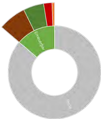
Wärmeerzeugung 2016 in %
