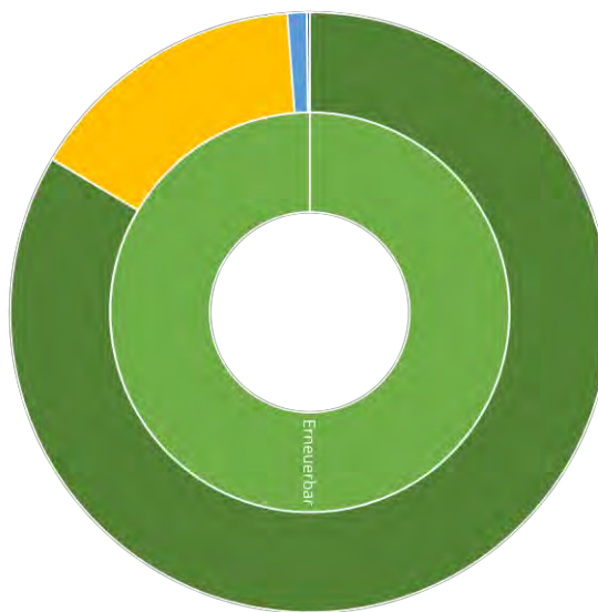
Stromerzeugung 2016 in %
