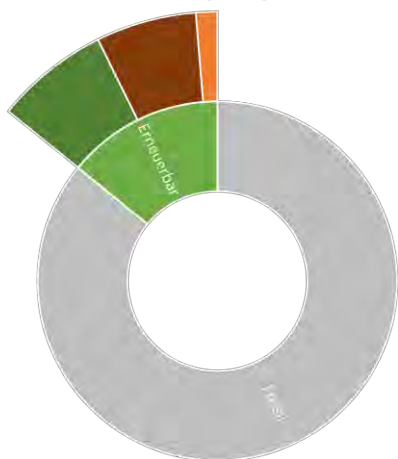
Wärmeerzeugung 2016 in %
